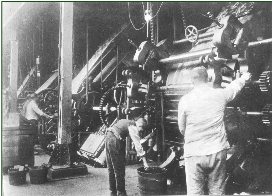
De roldrukkerij bij van Vlissingen te Helmond omstreeks 1900 waar zeven van deze machines, elk aangedreven door een stoommachine stonden. De grootste had een snelheid van 8 meter per minuut met een hoofdas van meer dan 5 meter.
